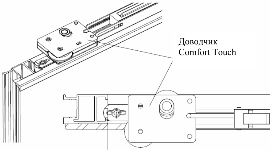
Правильно установленный в горизонтальный верхний профиль Доводчик Comfort Touch
