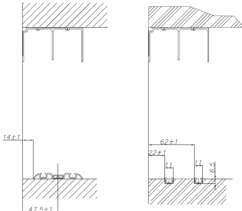
Положение нижней рельсы
